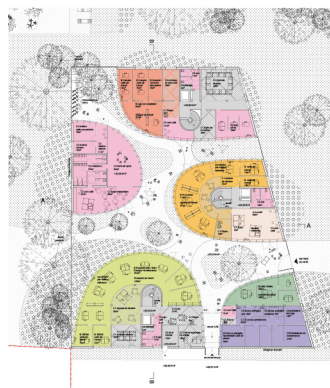
Plan du B2C-1/200
