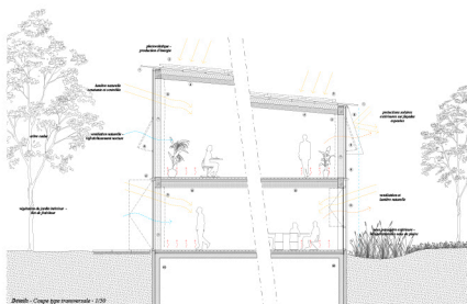
Coupe type transversale du bâtiment d'exploitation
