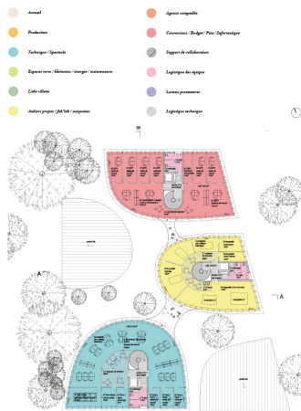
Plan du B1-1/200
