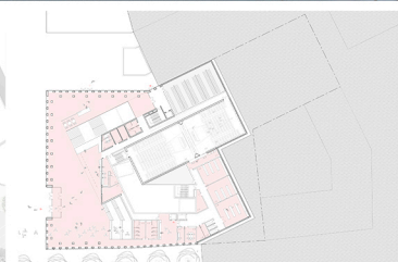
PLAN DÉTAILLÉ - ECH 1/500
