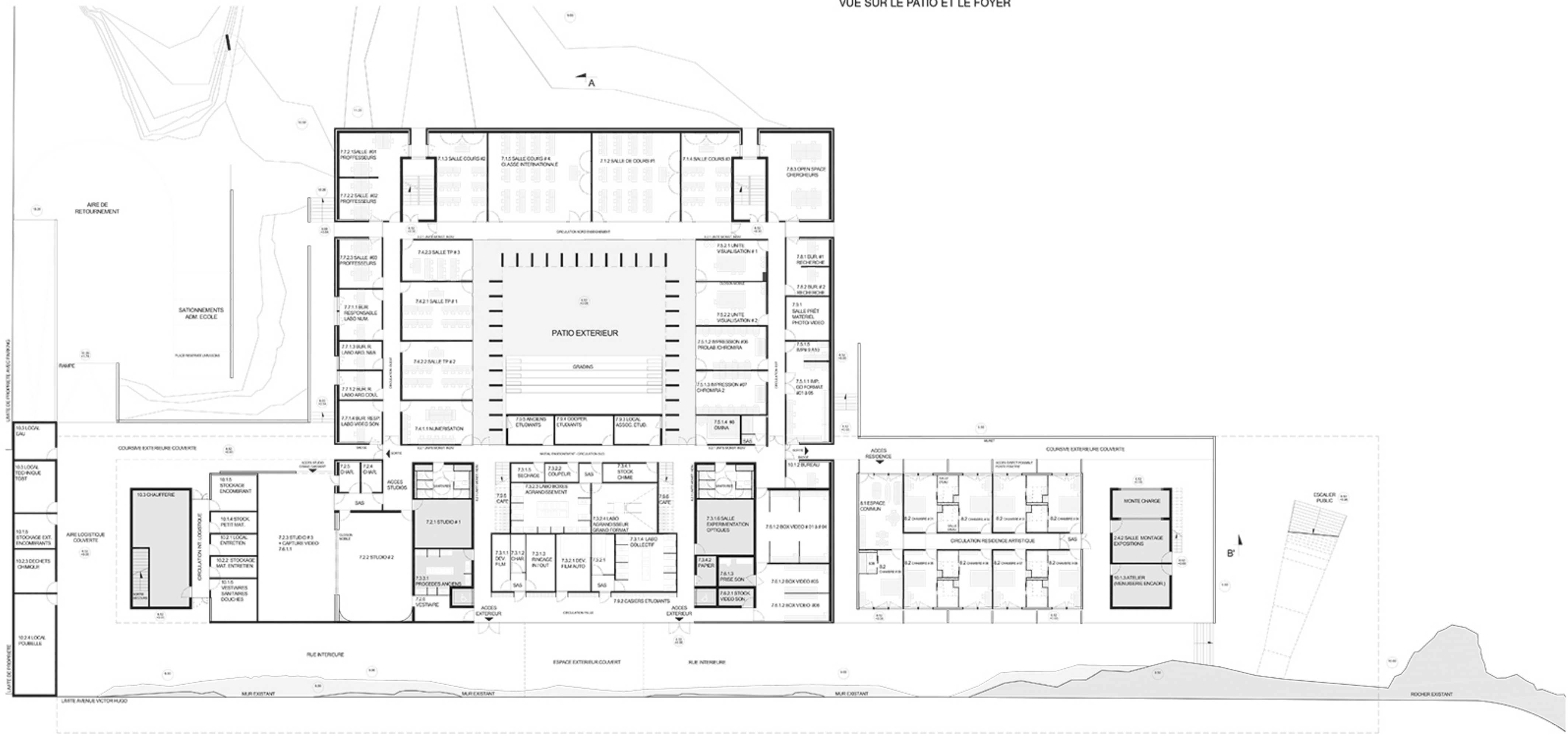
PLAN DU REZ-DE-JARDIN (NIVEAU 0) 1/200 ème
