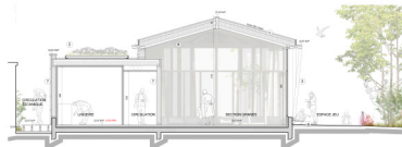
COUPE TRANSVERSALE BB 1/50
