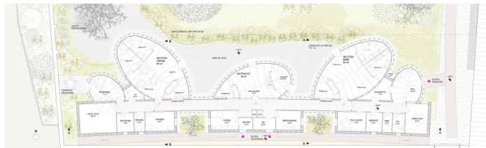
PLAN RDC 1/100
