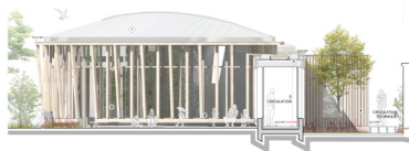
COUPE TRANSVERSALE AA 1/50
