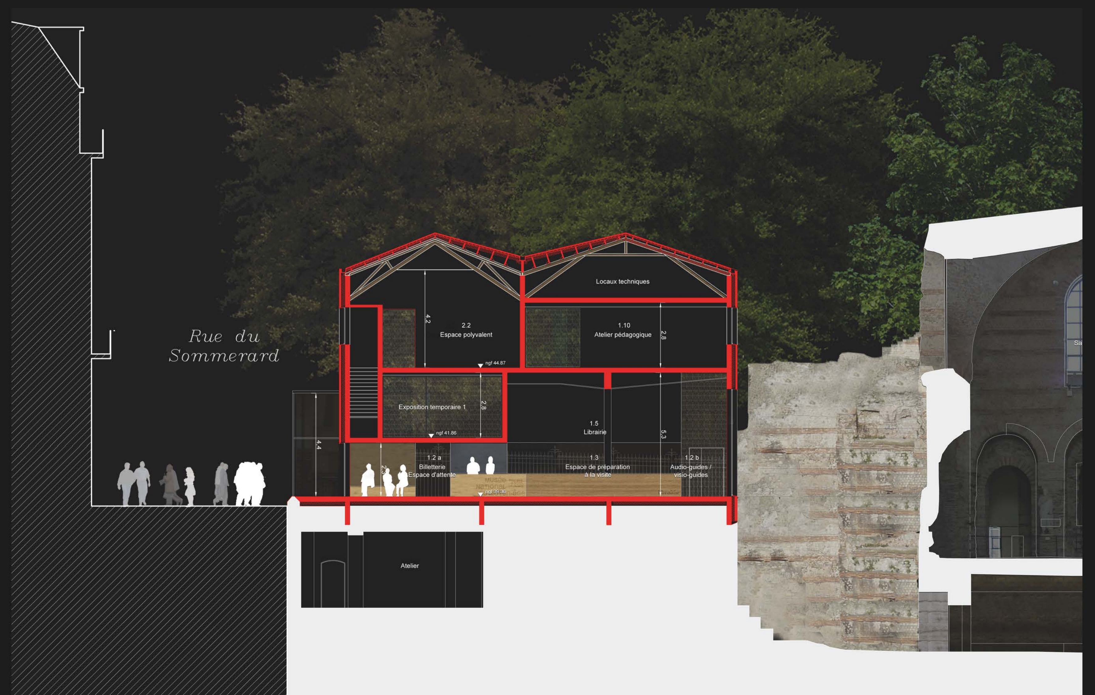
COUPE DD 1/100
